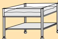
MOBILNI PESKOVNIK s pleksi koritom in sp. poličko 90 x 60
