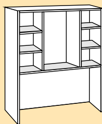
IGRALNI KOTIČEK FRIZERSKI / LN 120/IKF 90 x 40 x 120
