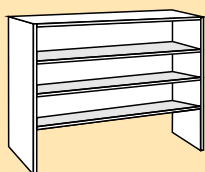
OMARA OBZIDNA / LN 2/120-O/PR/Z s policami in prostorom za mobilne predale 90 x 40 x 120
